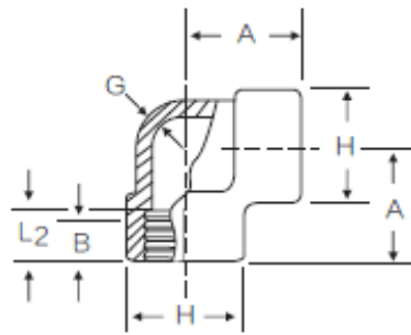
90°弯头90°ELBOW
