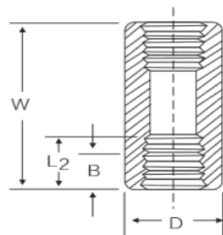
双承口管箍COUPLING
